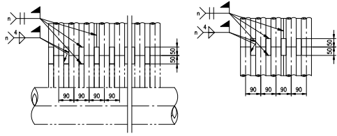
顺式壁与集管侧角钢连接详图 1:10
