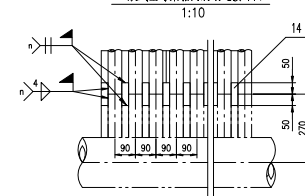
膜式壁与集箱间扁钢连接详图
