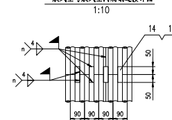
膜式壁与膜式壁间扁钢连接详图
